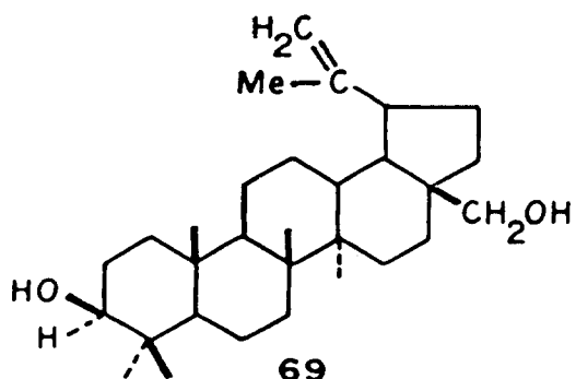
Betulin
