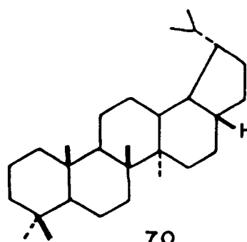
17β(H) 28-norlupane
