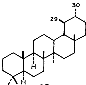
Ursane
