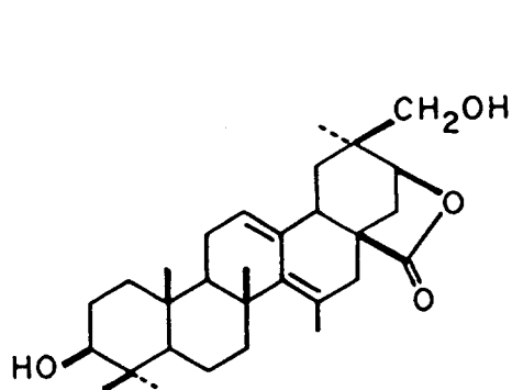
39 Pachanol
