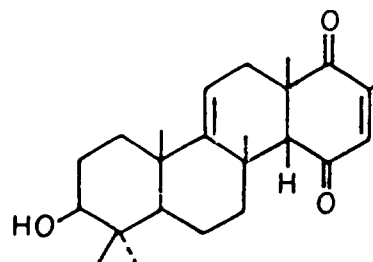
Isoarborneol
