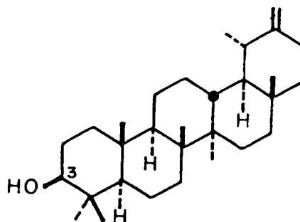
Taraxastane
