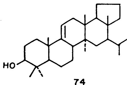
Isoarborneol
