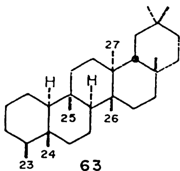
Friedelane
