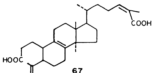
Manwuweizic acid
