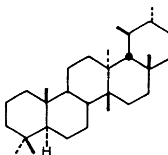
Bauerane
